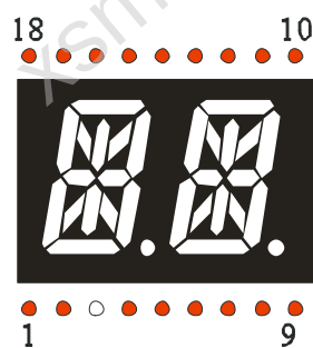
数码管显示及引脚位置图 3 NO PIN
