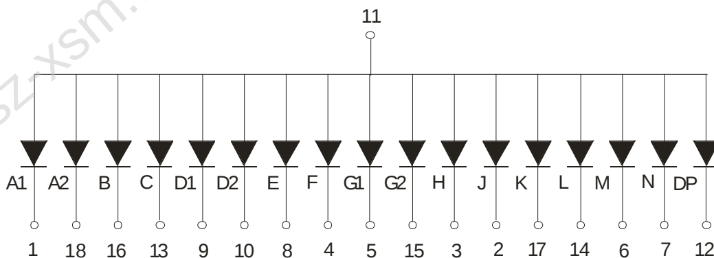
数码管显示及引脚位置图
