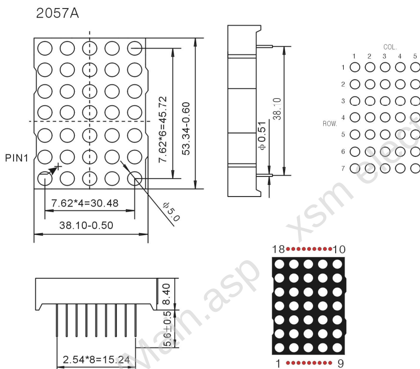
数码管显示及引脚位置图
