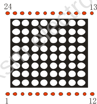
数码管显示及引脚位置图
