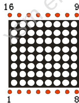
数码管显示及引脚位置图
