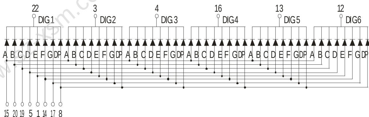
数码管显示及引脚位置图 2,6,7,9,10,11,18,21 NOPIN
