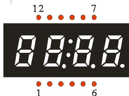
数码管显示及引脚位置图
