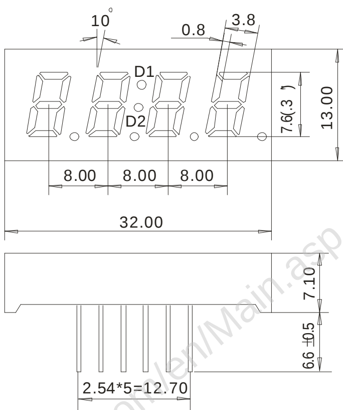
数码管显示及引脚位置图
