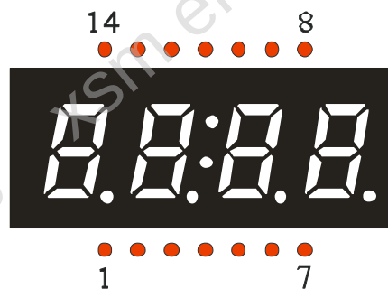
数码管显示及引脚位置图
