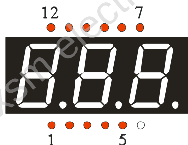
数码管显示及引脚位置图 6 NO PIN
