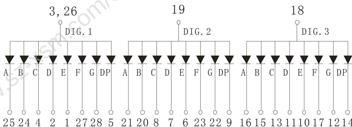
数码管显示及引脚位置图
