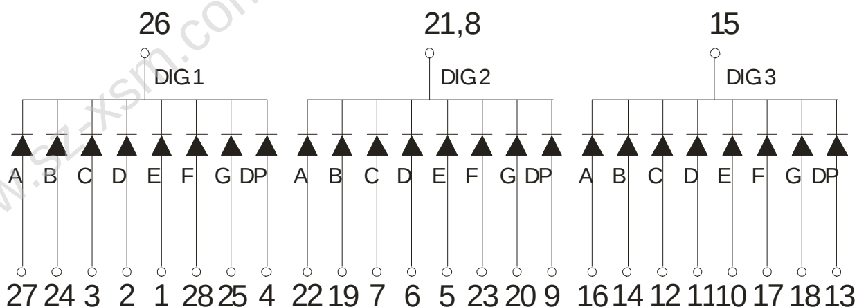
数码管显示及引脚位置图
