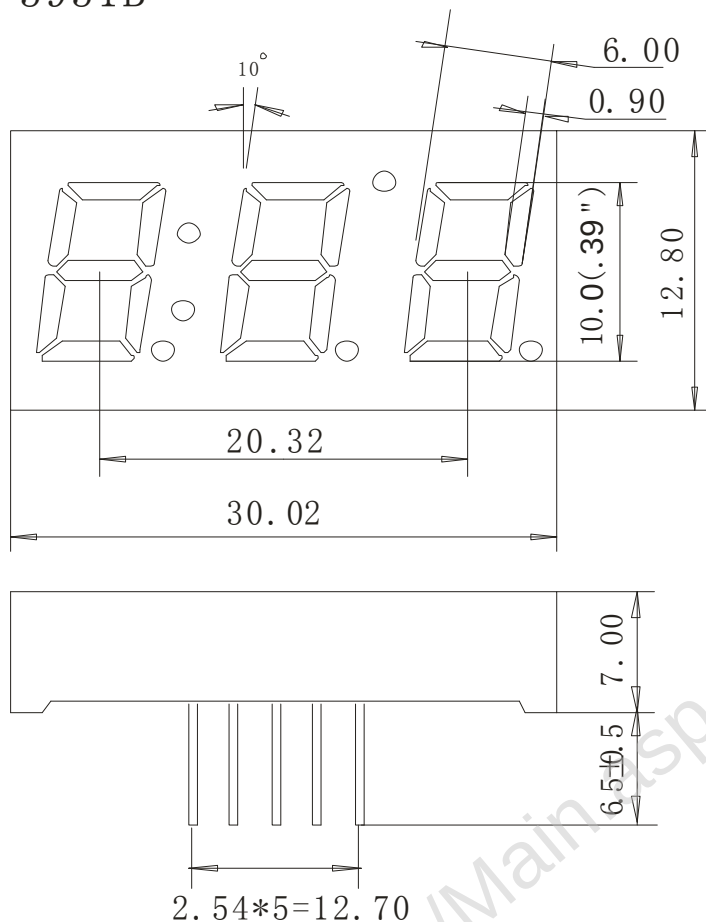
数码管显示及引脚位置图 6 NO PIN
