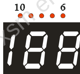
数码管显示及引脚位置图
