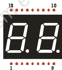
数码管显示及引脚位置图
