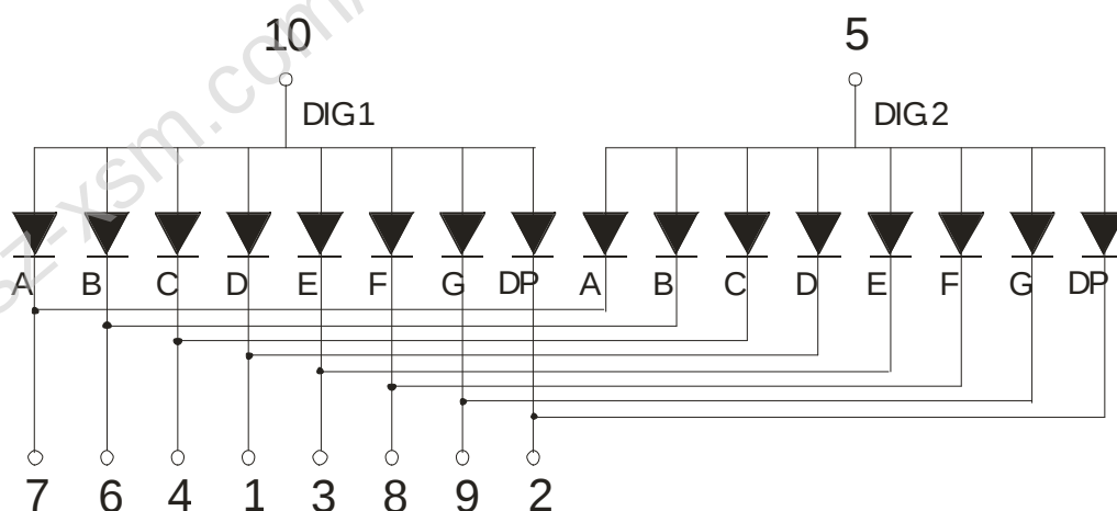
数码管显示及引脚位置图
