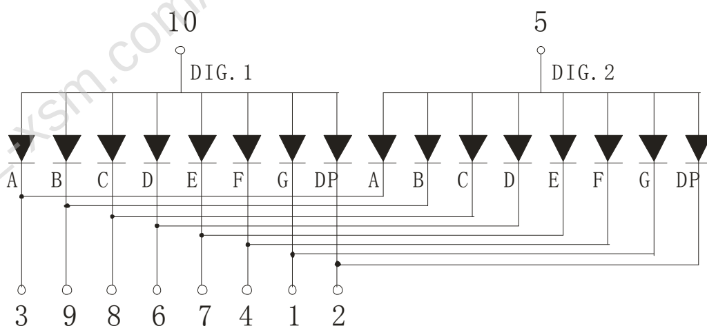
数码管显示及引脚位置图
