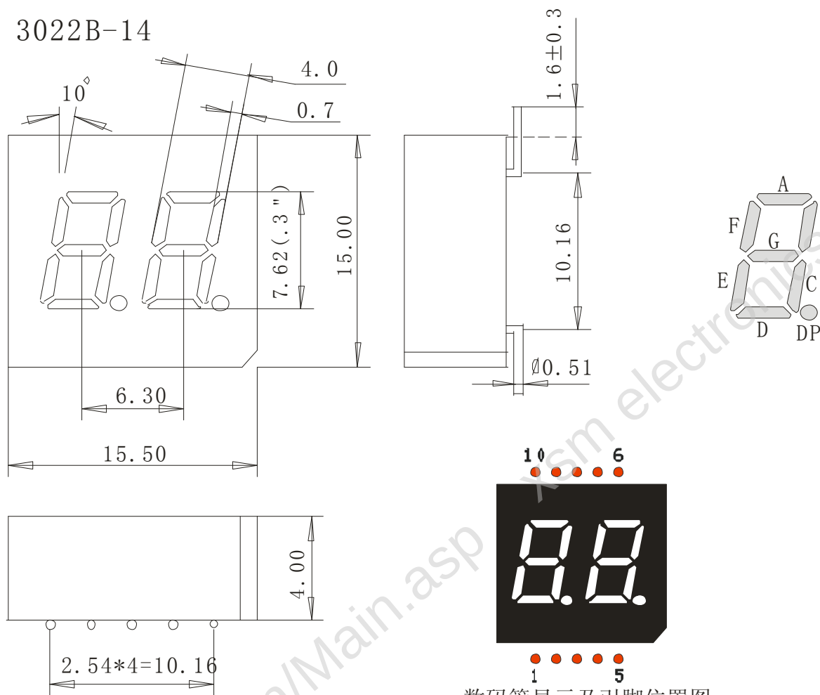
数码管显示及引脚位置图
