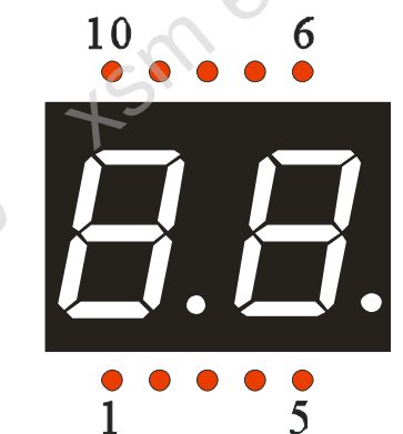
数码管显示及引脚位置图
