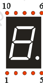
数码管显示及引脚位置图
