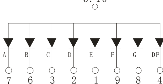
数码管显示及引脚位置图
