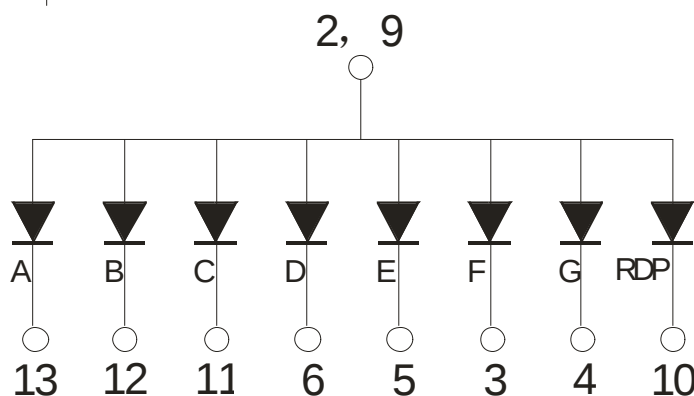
数码管显示及引脚位置图 1, 7, 8, 14 NOPIN
