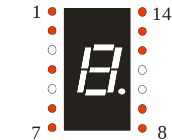
数码管显示及引脚位置图 3, 5, 10, 11 NOPIN
