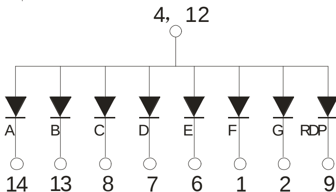
数码管显示及引脚位置图 3, 5, 10, 11 NOPIN
